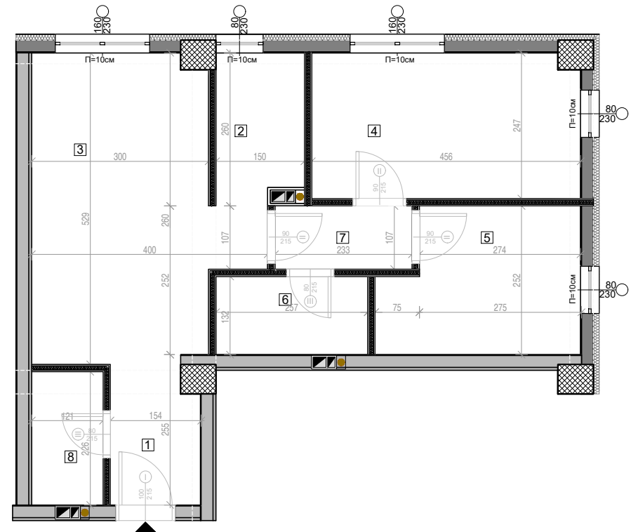
ТЕХНИЧКА ОСНОВА СО ДИМЕНЗИИ
