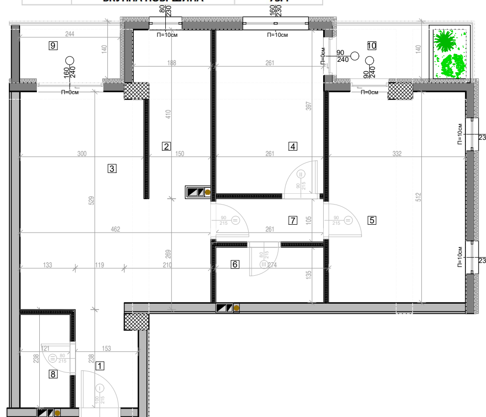
ТЕХНИЧКА ОСНОВА СО ДИМЕНЗИИ
