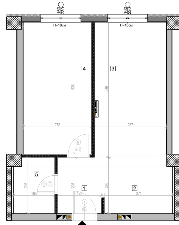
ТЕХНИЧКА ОСНОВА СО ДИМЕНЗИИ
