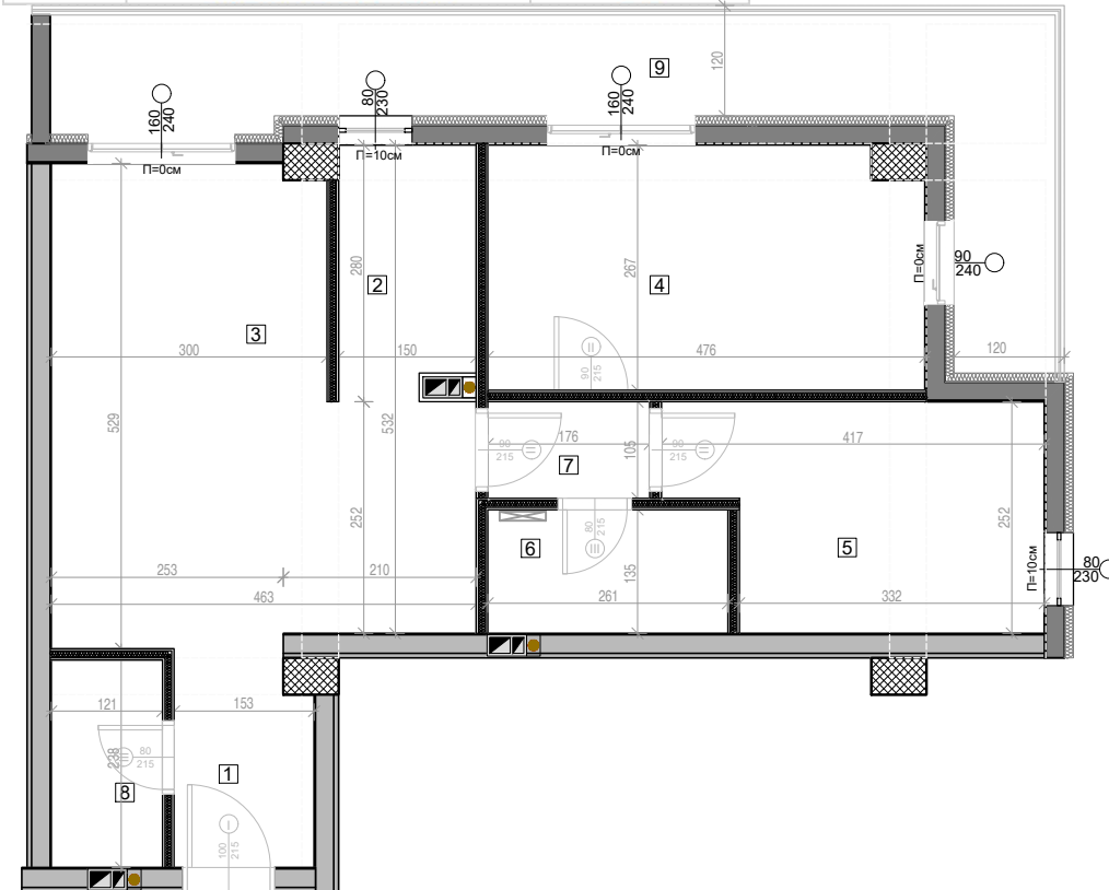
ТЕХНИЧКА ОСНОВА СО ДИМЕНЗИИ
