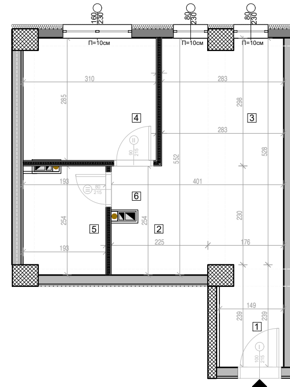
ТЕХНИЧКА ОСНОВА СО ДИМЕНЗИИ
