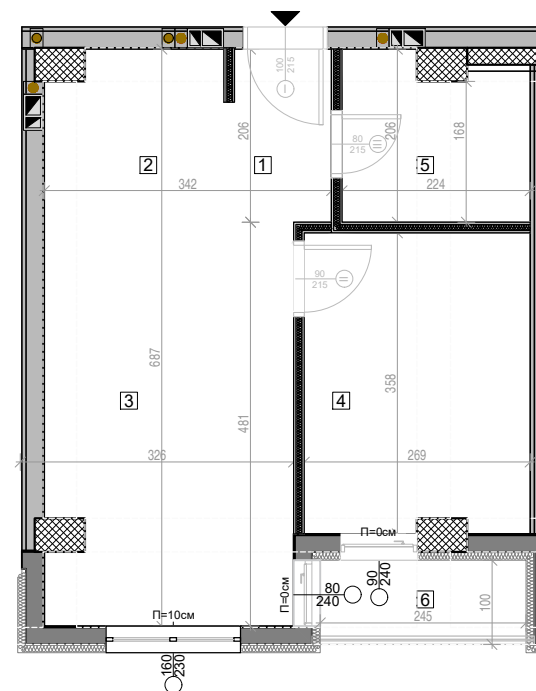
ТЕХНИЧКА ОСНОВА СО ДИМЕНЗИИ
