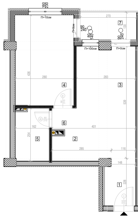
ТЕХНИЧКА ОСНОВА СО ДИМЕНЗИИ
