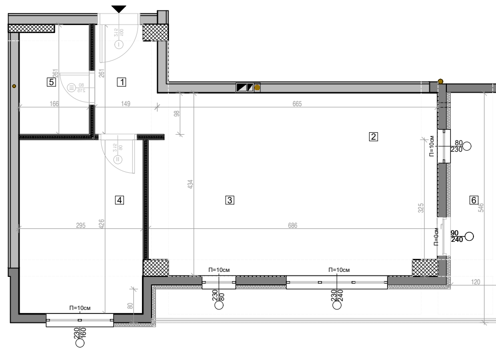
ТЕХНИЧКА ОСНОВА СО ДИМЕНЗИИ
