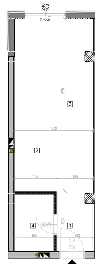
ТЕХНИКА ОСНОВА СО ДИМЕНЗИИ
