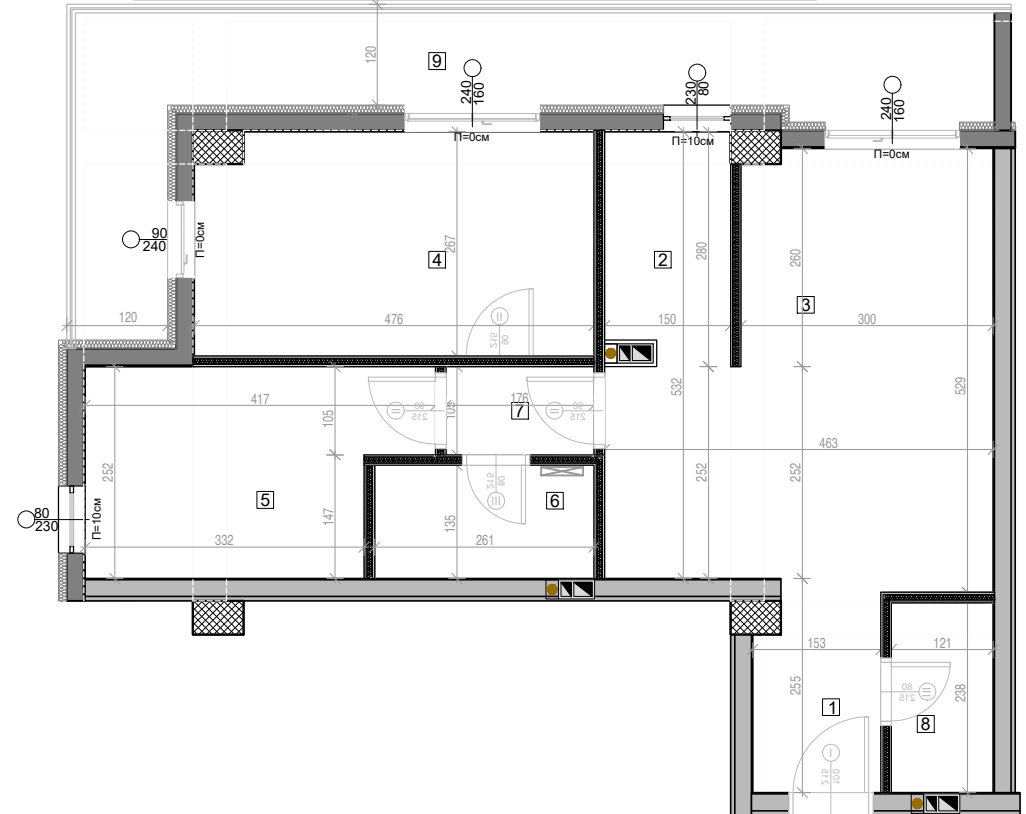
ТЕХНИЧКА ОСНОВА СО ДИМЕНЗИИ
